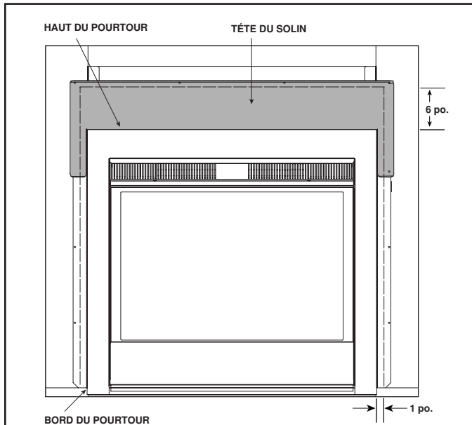
Figure 7.5 Vue de l'extérieur sans le revêtement primaire non combustible
