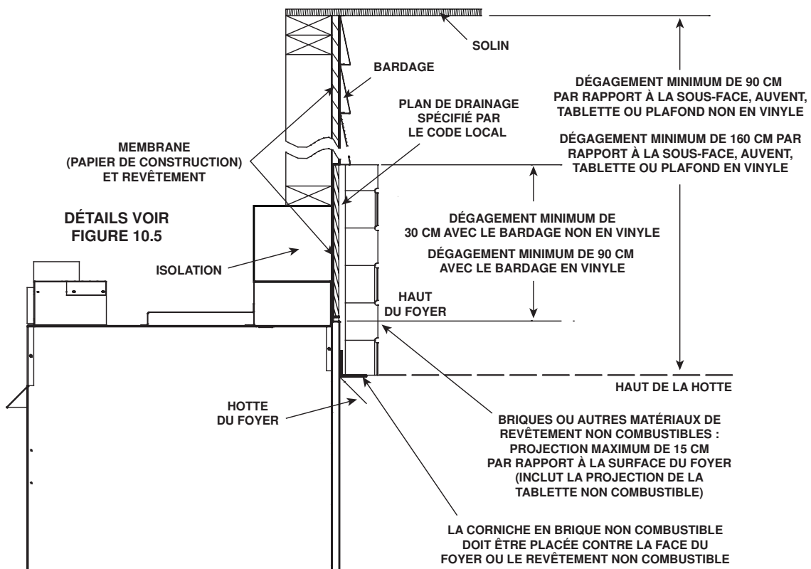
Figure 10.7 Vue extérieure du revêtement décoratif non combustible
