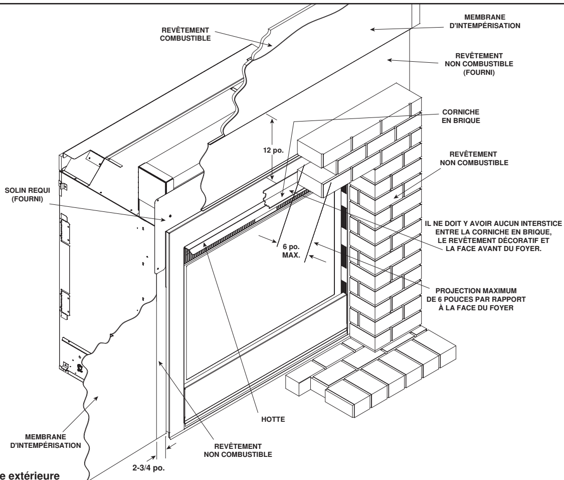
Figure 10.5 Vue extérieure
