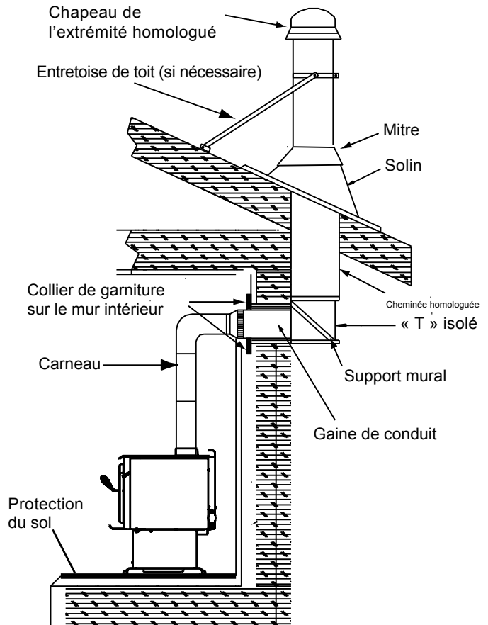
Figure 12.1 Cheminée préfabriquée pour l'extérieur
