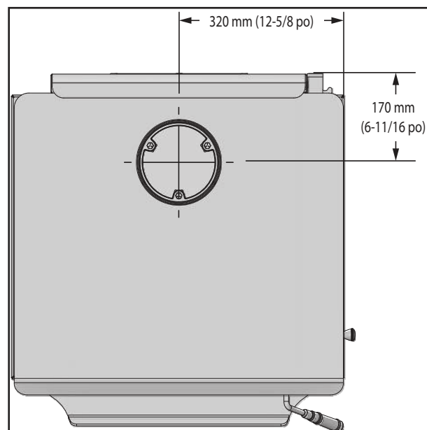
Figure 7.2 Vue de dessus
