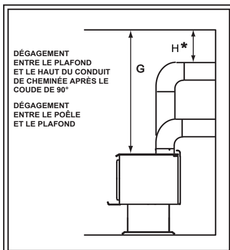
INSTALLATION DANS UN COIN
