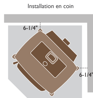
Installation en coin Protection plancher en coin 36" x 36" minimum
