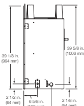
Vue latérale droite
