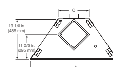
Vue en plan
