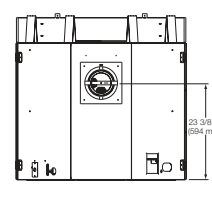
Vue arrière
