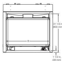
Vue frontale
