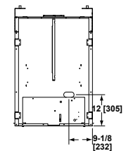
VUE LATÉRALE
