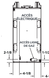
VUE LATÉRALE
