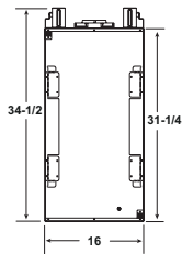
VUE LATÉRALE
