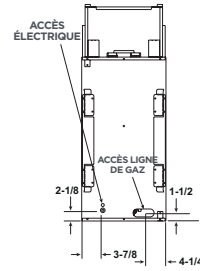
VUE LATÉRALE
