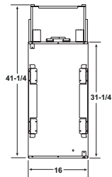
VUE LATÉRALE
