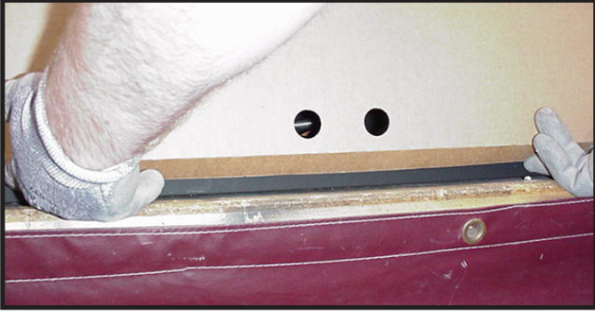
Figure 13.6 Pliage du rabat inférieur
