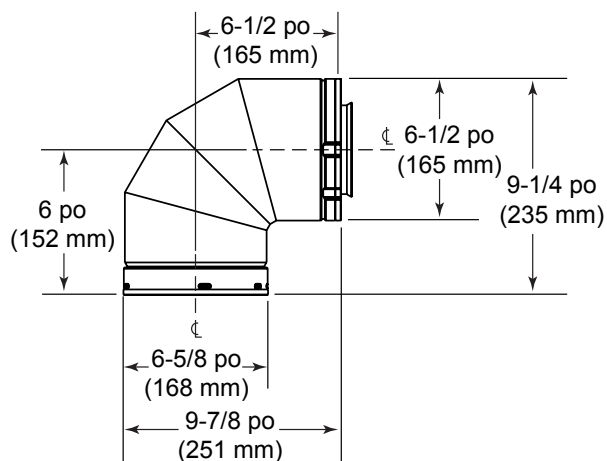
SLP90 Coude de 90°
