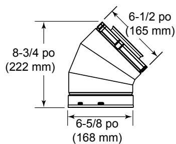
SLP45 Coude de 45°
