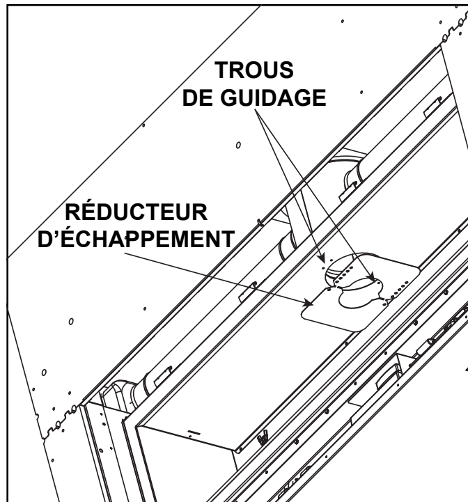
Figure 4.9 Réducteur d'échappement
