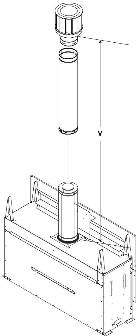
Figure 4.8 Conduit maximal d'évacuation verticale
