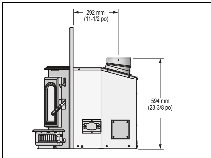
Figure 8.1 - Vue latérale avec l'adaptateur à 15 degrés optionnel
