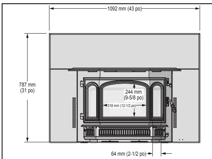
Figure 7.3 – Vue frontale - Petit encadrement d'acier
