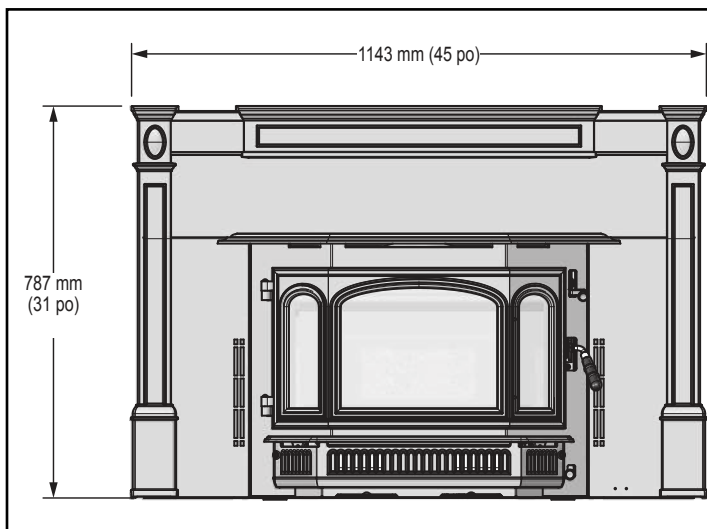
Figure 7.5 – Vue frontale - Petit encadrement de fonte
