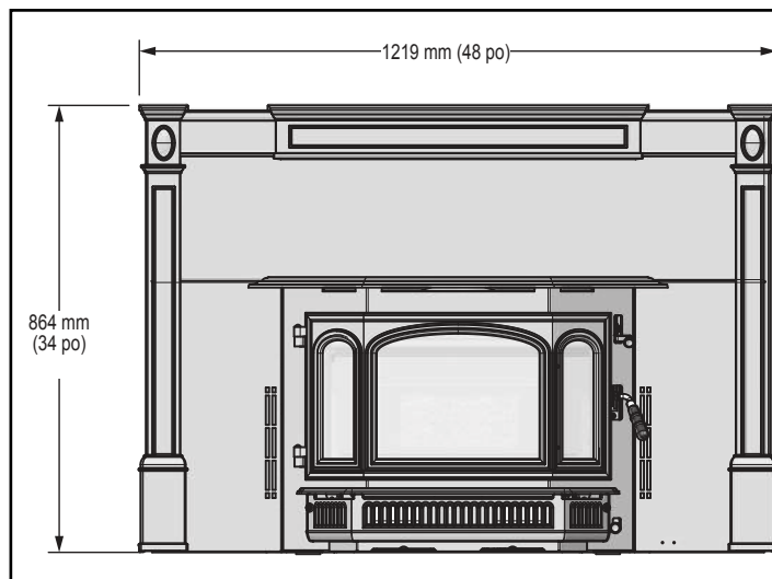
Figure 7.6 – Vue frontale - Grand encadrement de fonte
