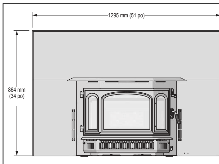
Figure 7.4 – Vue frontale - Grand encadrement d'acier
