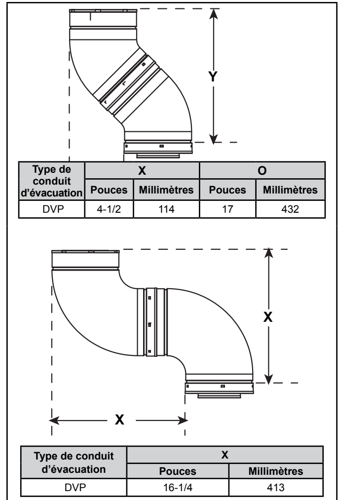
La figure 4.5 présente les dévoiements verticaux et horizontaux pour les coudes DVP.
