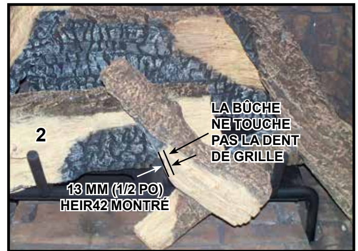
Figure 13. Disposition de la bûche n° 6
