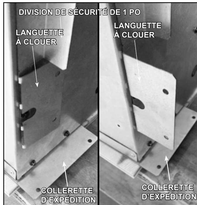
Figure 6.3 Languettes à clouer Position d'expédition
