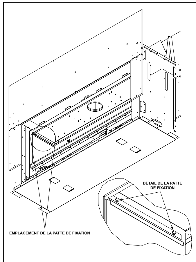
Figure 11.5 Installation de la patte de fixation – Modèles transparents
