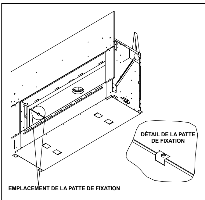
Figure 11.4 Installation de la patte de fixation – Modèles à un côté
