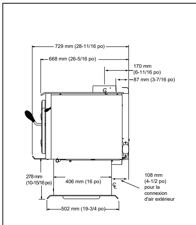
Figure 7.2 Vue latérale
