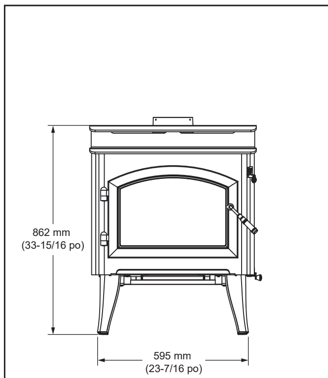
Figure 9.1 – Vue avant
