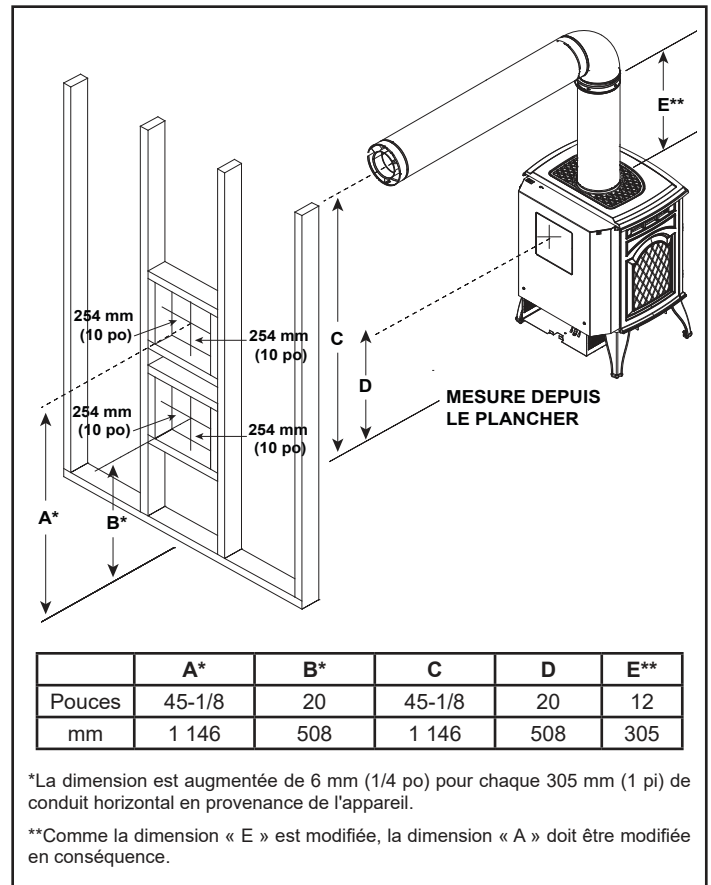
Figure 5.2 Pénétration d'un mur
