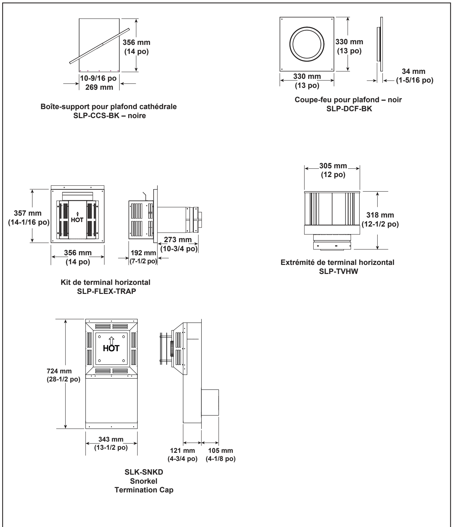
Figure 11.3 Composants du conduit de la série SLP
