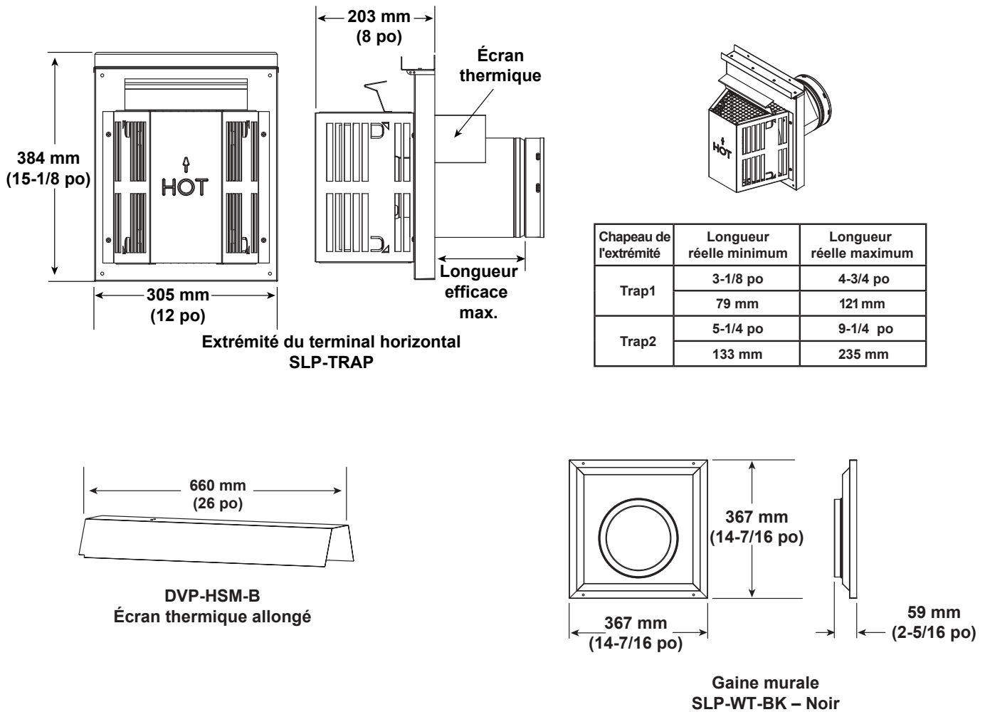
Figure 11.2 Composants du conduit de série SLP
