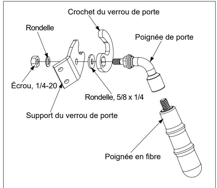
Figure 24.3 - Poignée de porte pour porte voûtée
