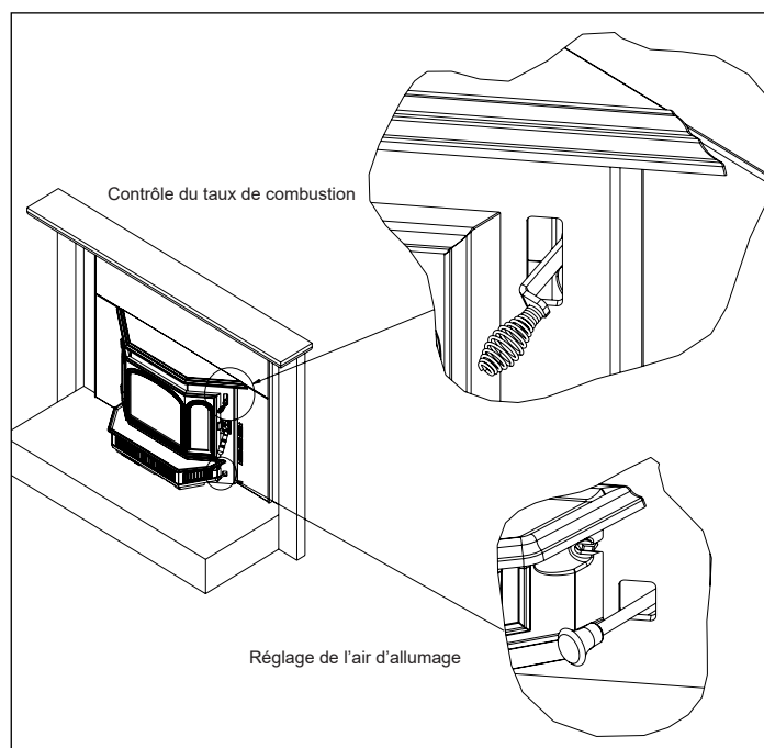
Figure 11.1 Réglages de l'air à l'allumage et de combustion
