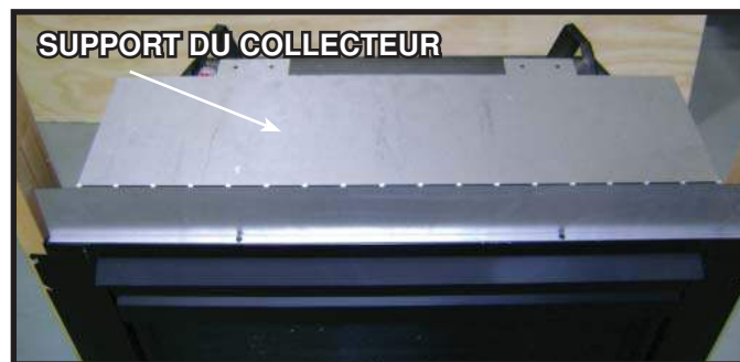
Figure 9.10 Plier le support du collecteur
