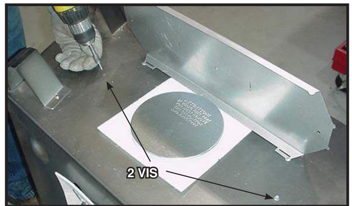
Figure 9.5 Remplacer les deux vis, tel qu'illustré.
