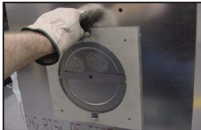
Figure 9.12 Plier les attaches du centre du tampon pare-feu (90°) vers l'intérieur et retirer le joint isolant.
