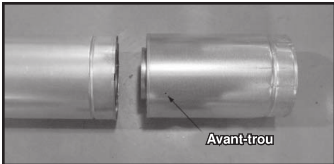
Figure 10.6 Avant-trous de la section coulissante
