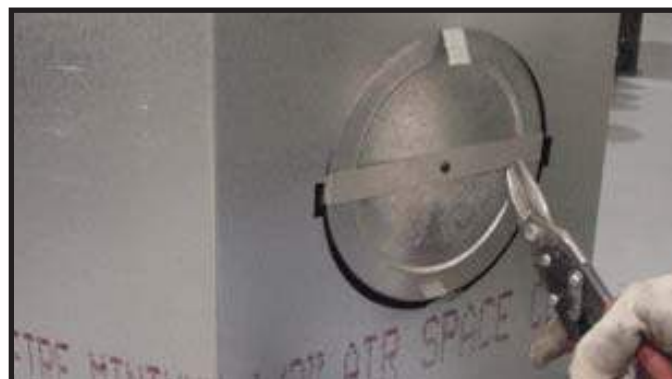
Figure 9.13 Coupez la bande de retenue en métal et pliez les bords vers l'extérieur.
