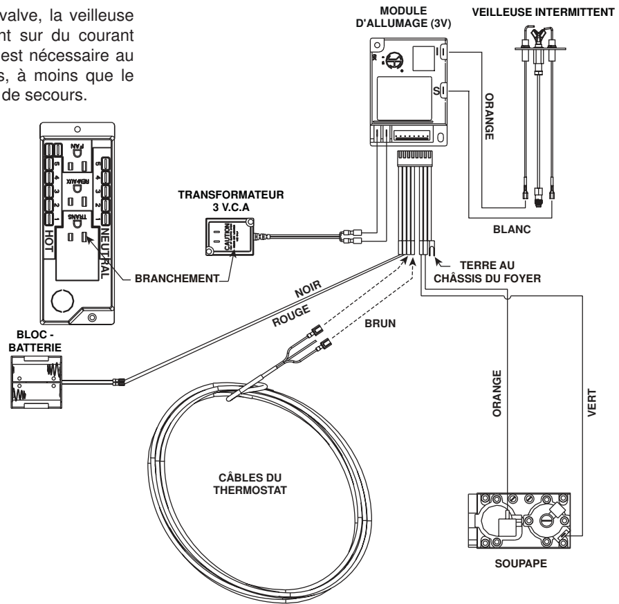
Figure 12.1 Diagramme de câblage de l'allumage à veilleuse Intellifire (IPI) avec un commutateur mural ou un thermostat
