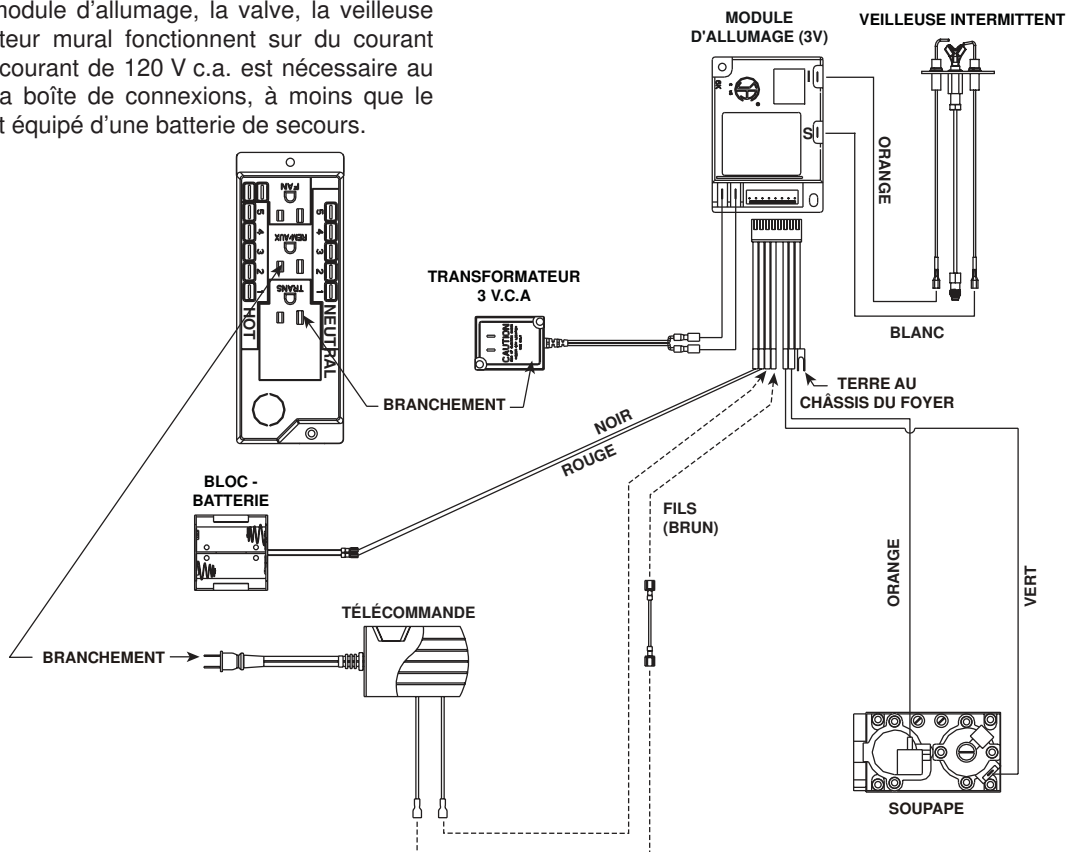
Figure 12.2 Diagramme de câblage de l'allumage à veilleuse Intellifire (IPI) avec une télécommande
