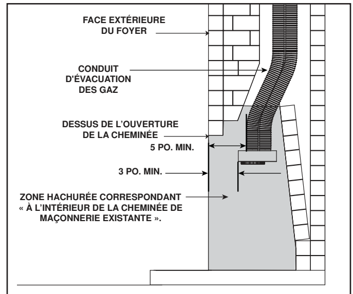
Figure 7.20 Foyer existant DV-46DVA-GCL, dégagements minimums
