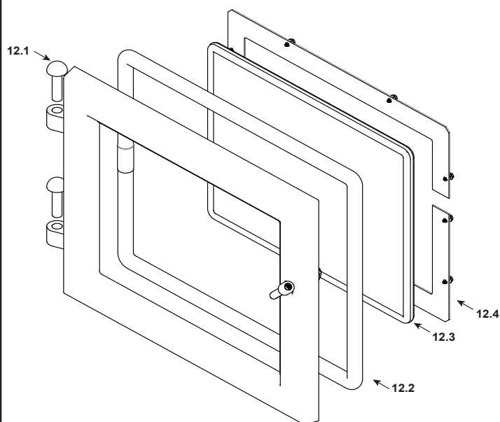
#12 Door Assembly
